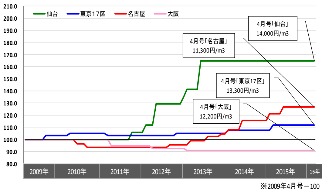
【図-3 全国主要都市における生コンクリートの価格推移】
