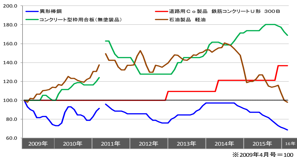
【図-1 仙台市における主要資材の価格推移】
